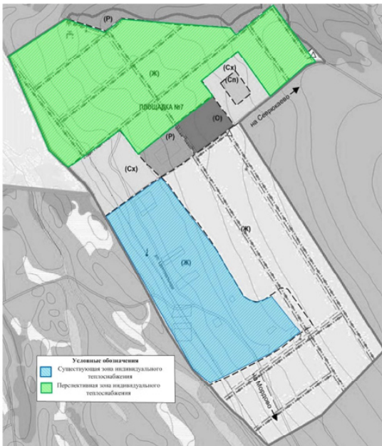
Рис. № 9 - Перспективные зоны действия индивидуального теплоснабжения на территории села Кольцово
