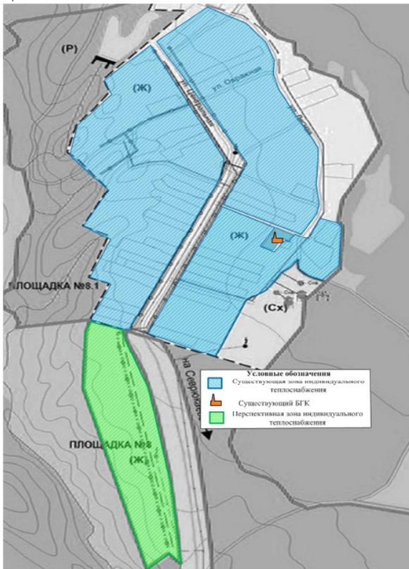
Рис. № 10 - Перспективные зоны действия индивидуального теплоснабжения на территории села Кармалы
