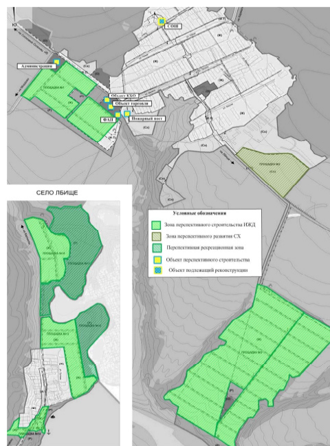
Рис. № 6 - Приросты строительных фондов, площадки и места перспективного строительства под жилую зону, а также размещение перспективных социально-значимых объектов на территории сел Севрюкаево и Лбиче
