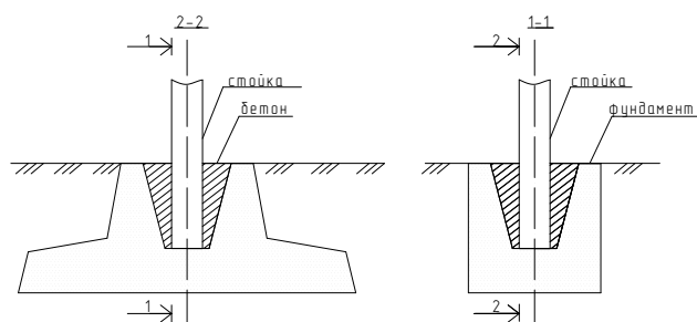
Рис. 1 Закрепление опор знаков в фундаменте
