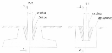
Рис. 1 Закрепление опор знаков в фундаменте
