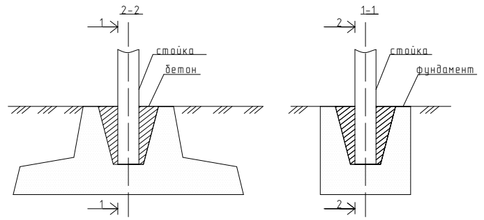
Рис. 1 Закрепление опор знаков в фундаменте
